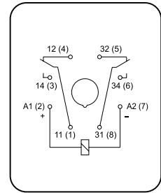
CR-U с 2 переключающими контактами
