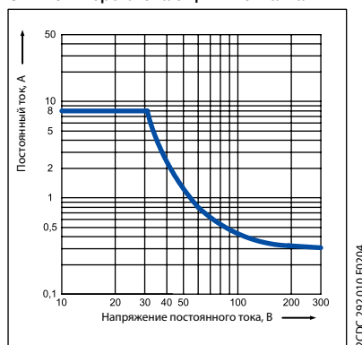
CR-P с 2 переключающими контактами
