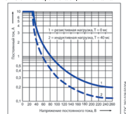
CR-U с 2 и 3 переключающими контактами
