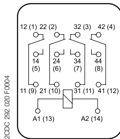
CR-M с 4 переключающими контактами
