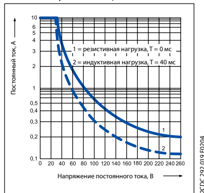
CR-M с 3 переключающими контактами
